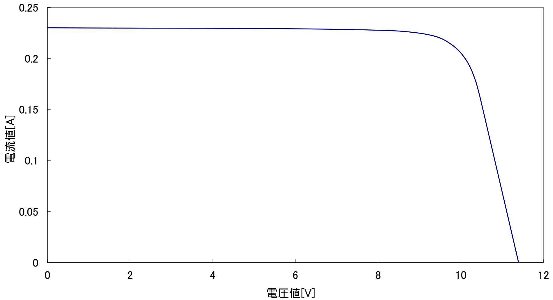
GT1618-MF 出力特性図 @1000W/m 2 AM1.5 25°C
