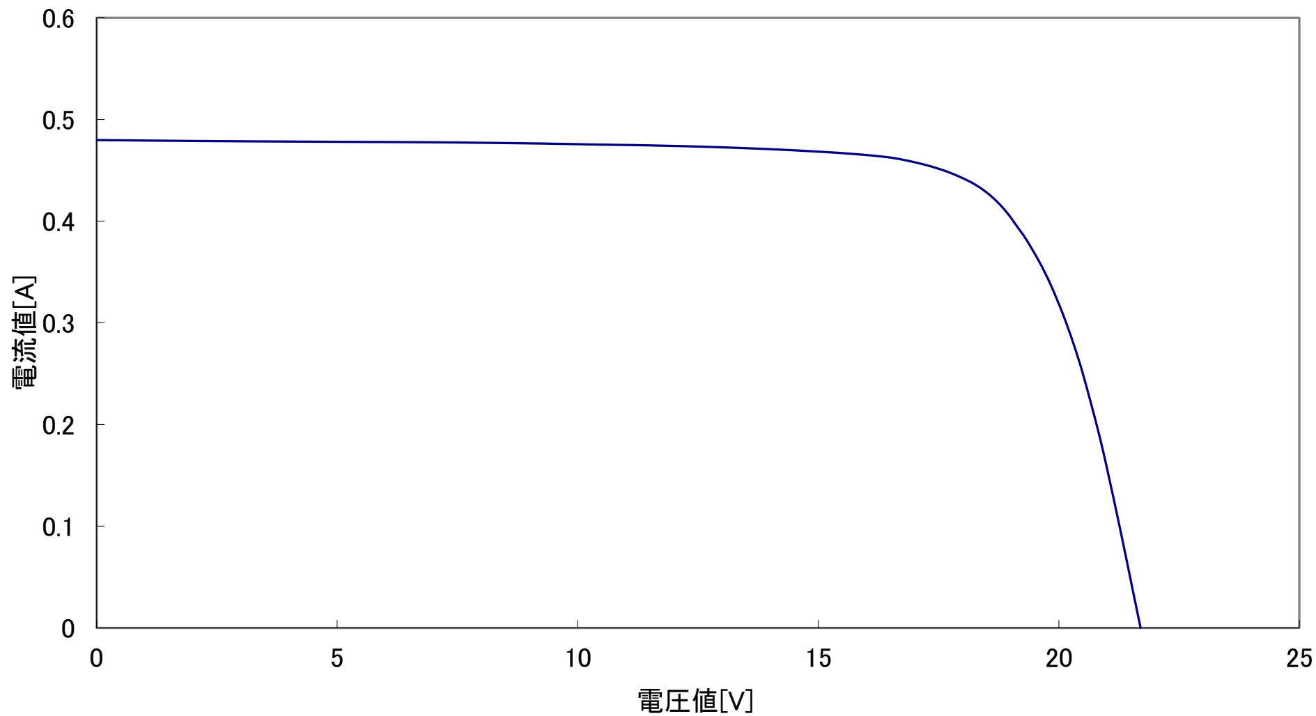
GT833S-TF 出力特性図 @1000W/m 2 AM1.5 25°C
