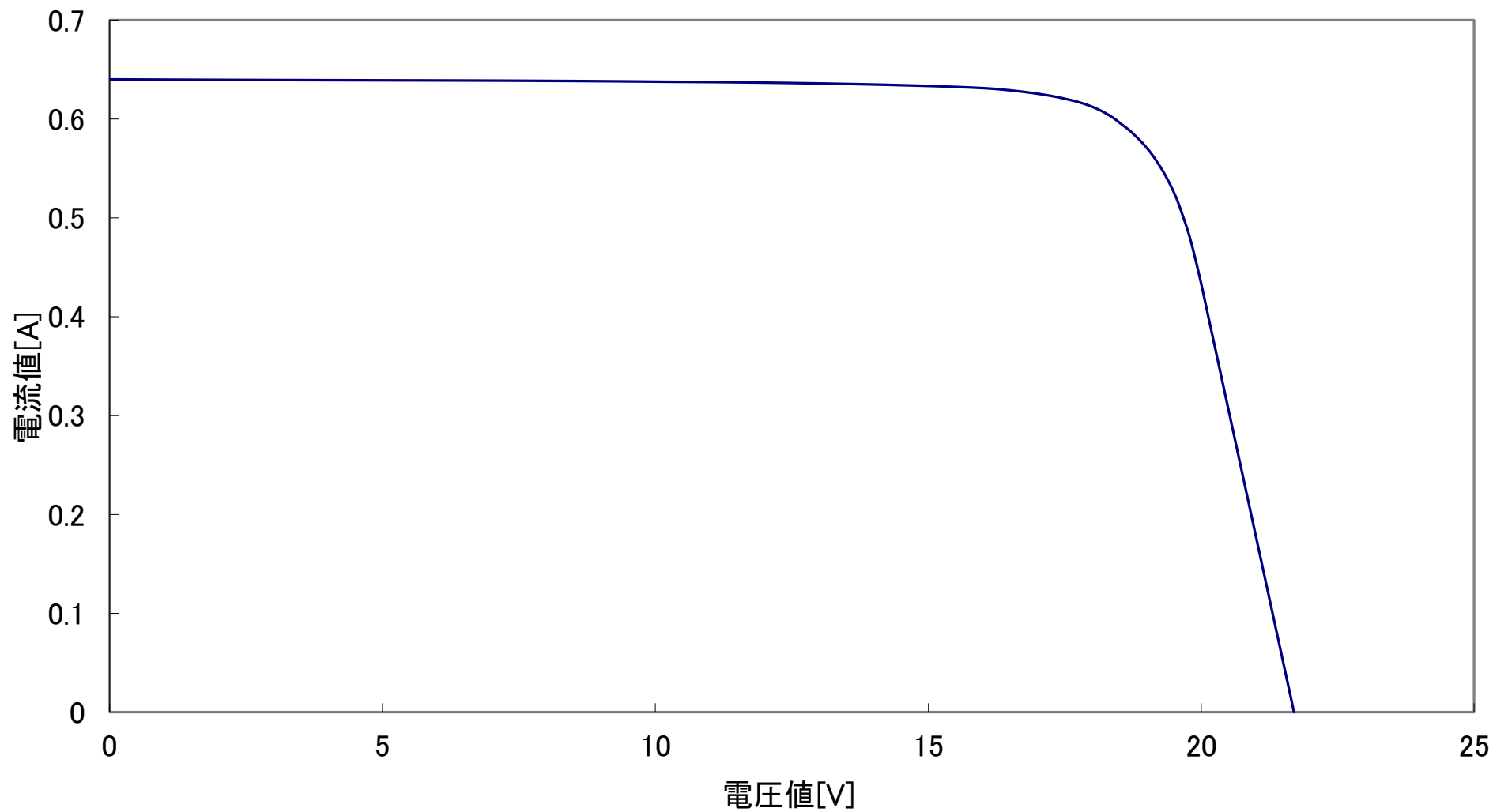
GT634 出力特性図 @1000W/m 2 AM1.5 25°C
