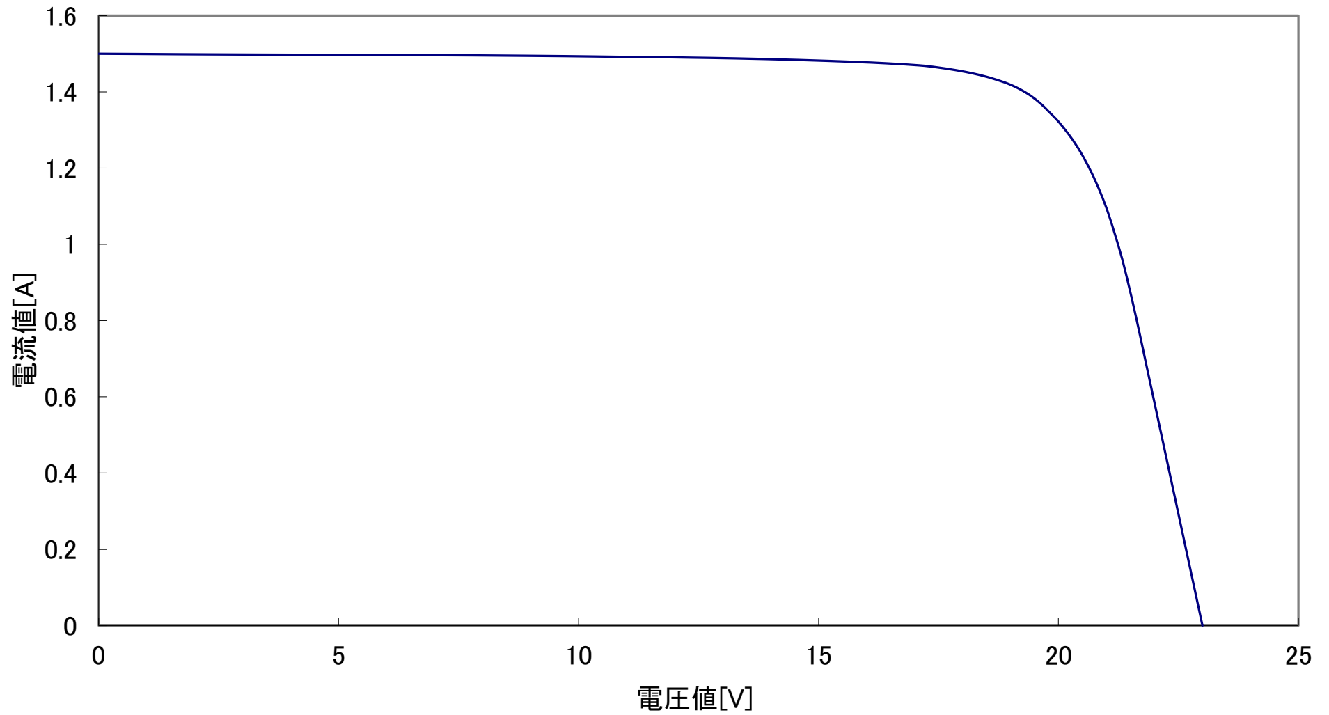
GT-K27 出力特性図 @1000W/m 2 AM1.5 25°C
