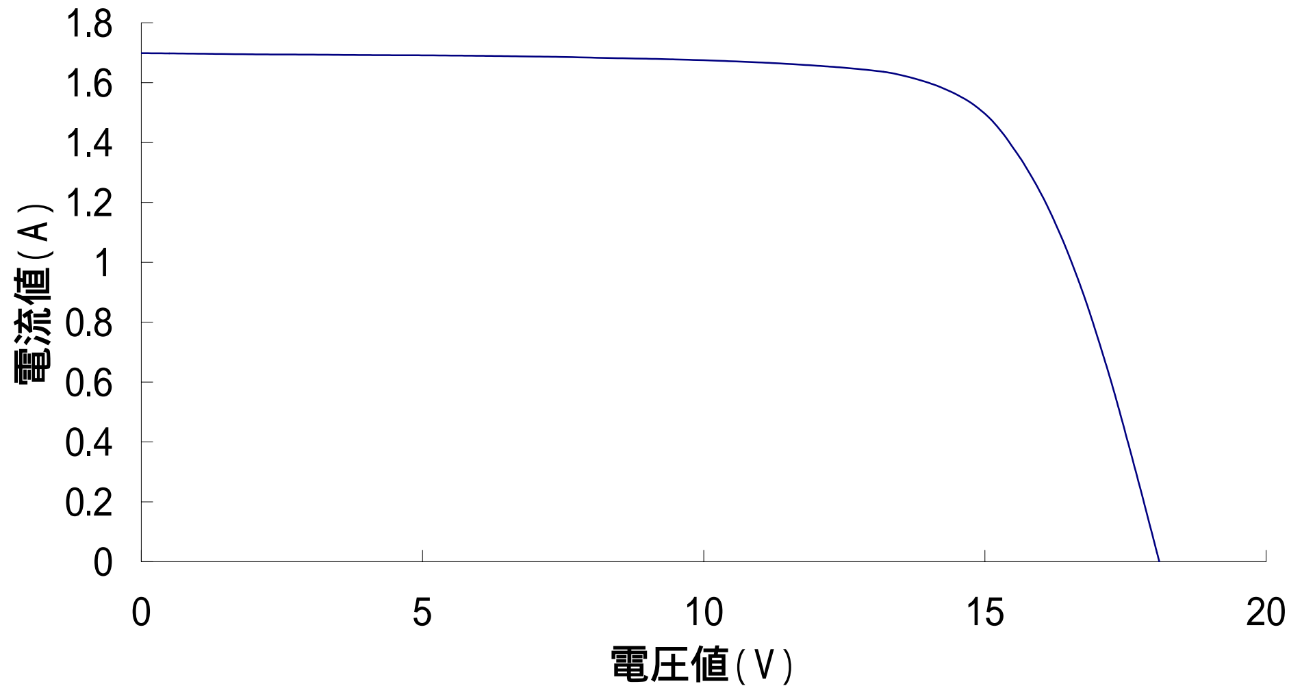
GT 2 3 0 出力特性図 @1000W/m 2 AM1.5 25
