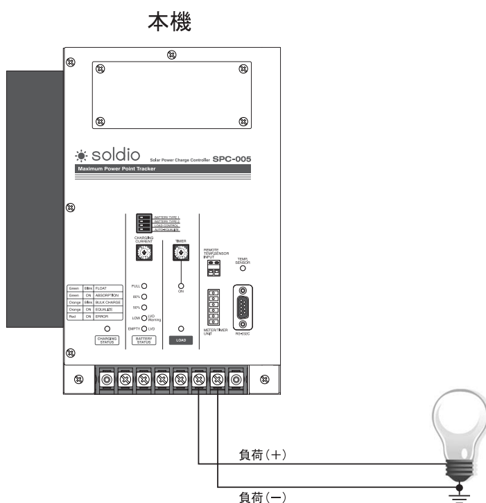
図 4.負荷配線
