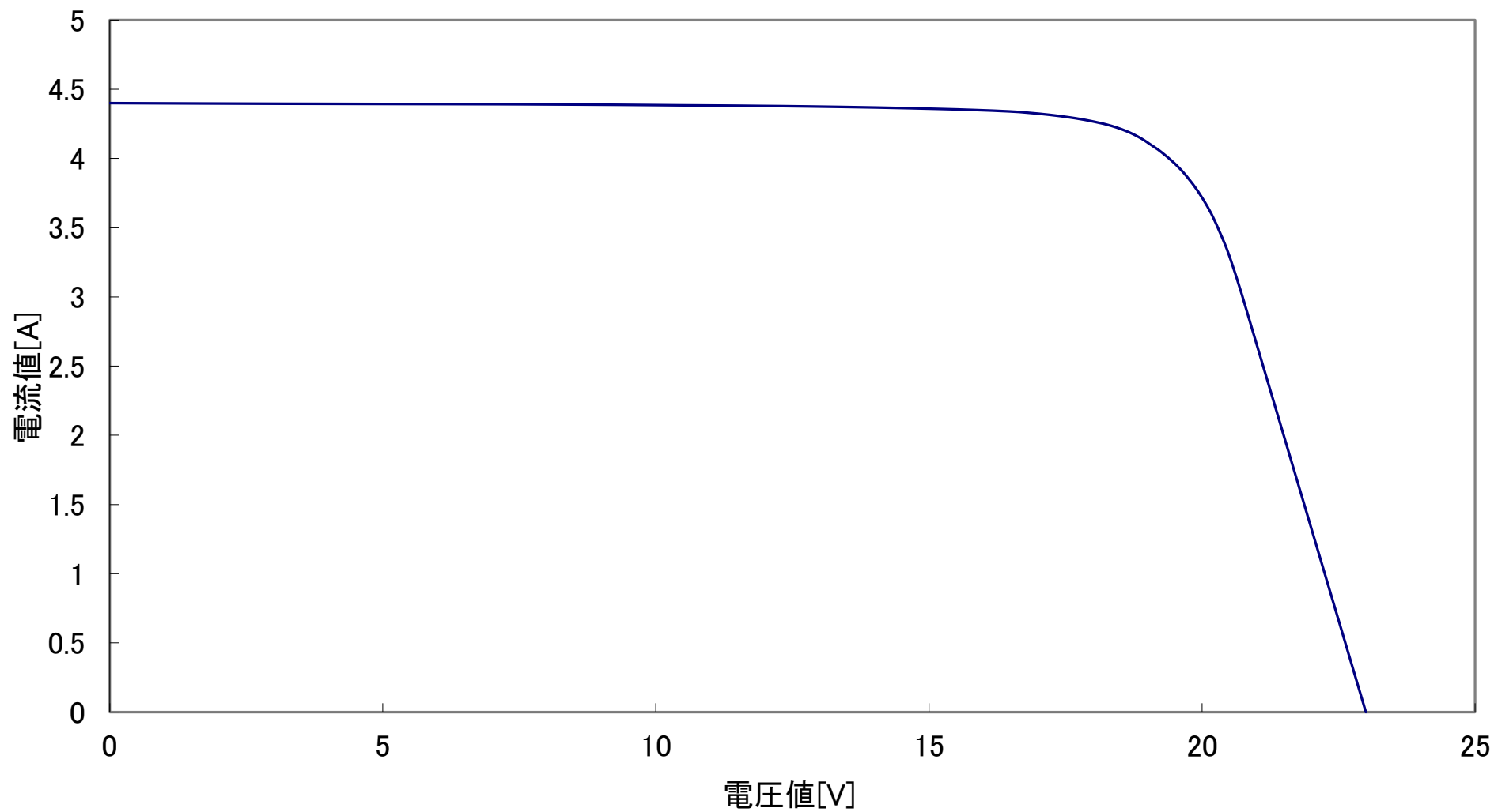
GT-K78 出力特性図 @1000W/m 2 AM1.5 25°C
